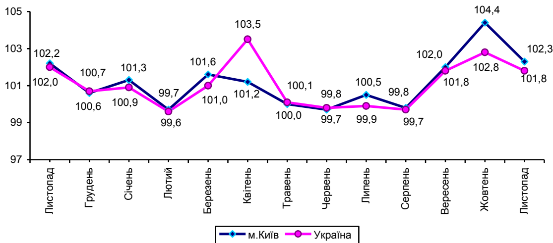
ІСЦ у 2015 - 2016 роках (у % до попереднього місяця)
